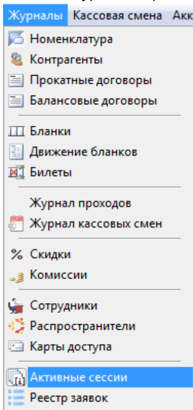
Рис.19.1.Активные сессии
