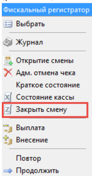
Рис.6.3.1.1. Закрытие фискальной смены
